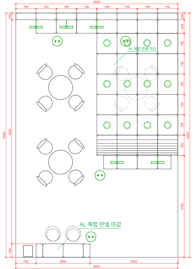
평면도 Scale: none
