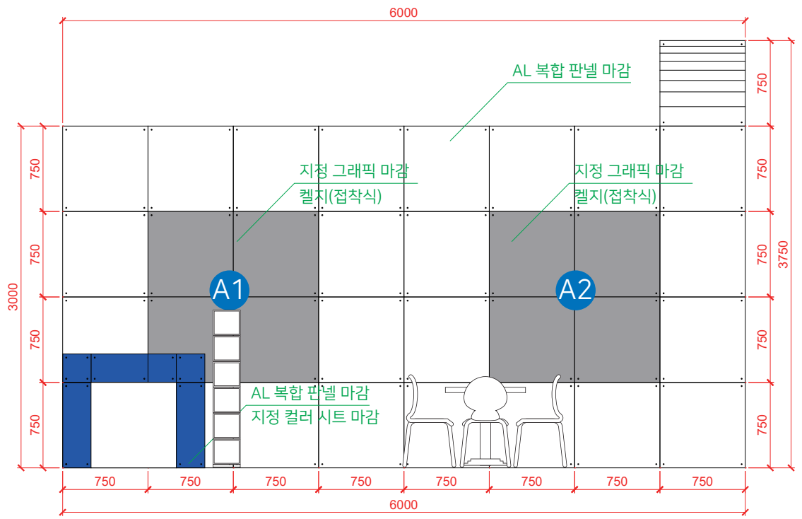
정면도 Scale: none
