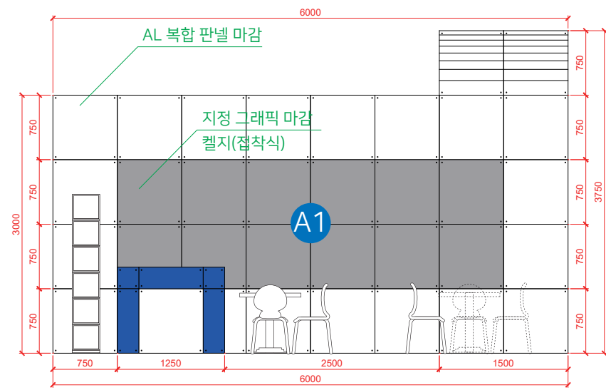
정면도 Scale: none
