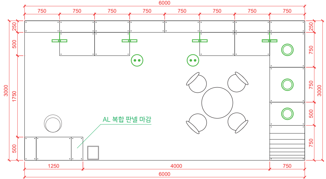
평면도 Scale: none
