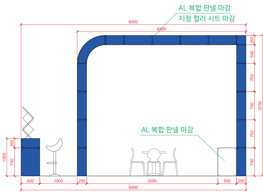
입면도(우) Scale: none
