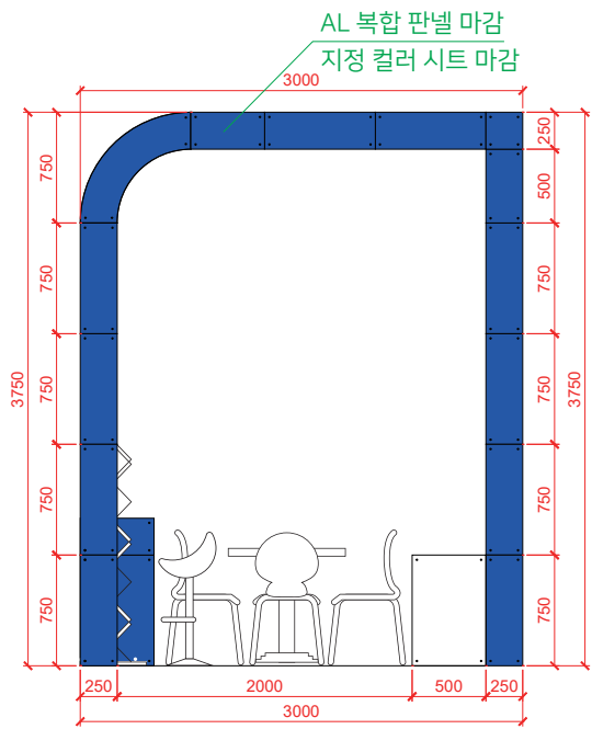
입면도(우) Scale: none
