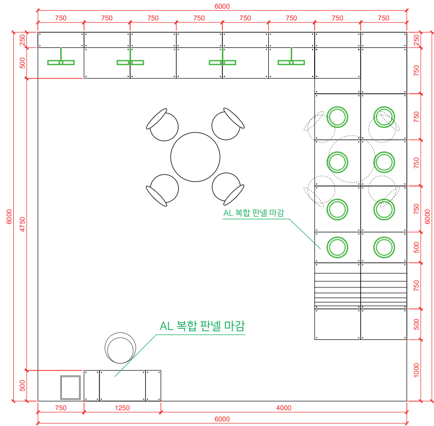
평면도 Scale: none
