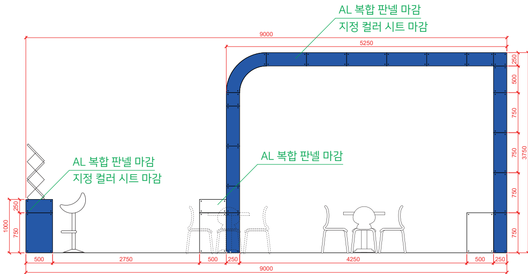
입면도(좌) Scale: none
