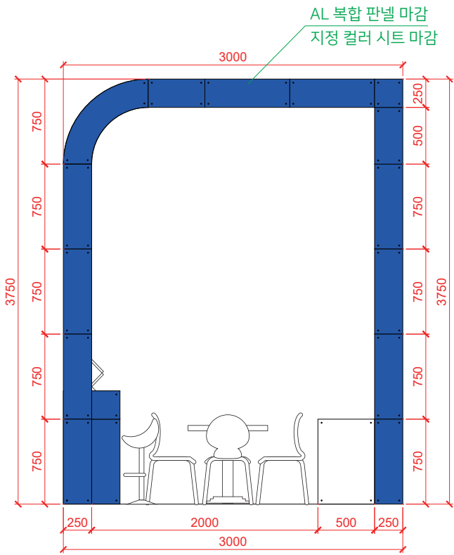
입면도(우) Scale: none
