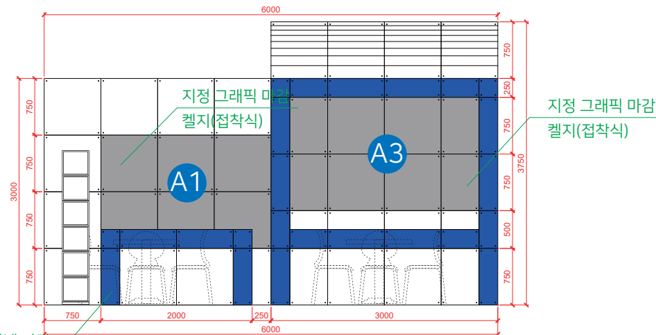
정면도 Scale: none
