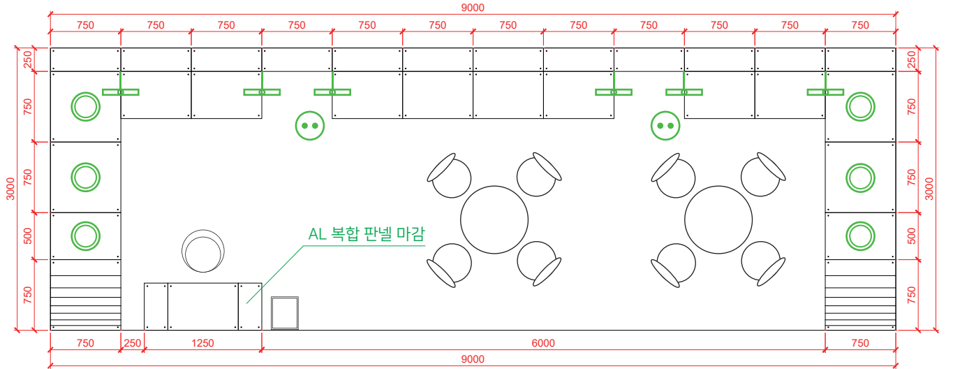
평면도 Scale: none
